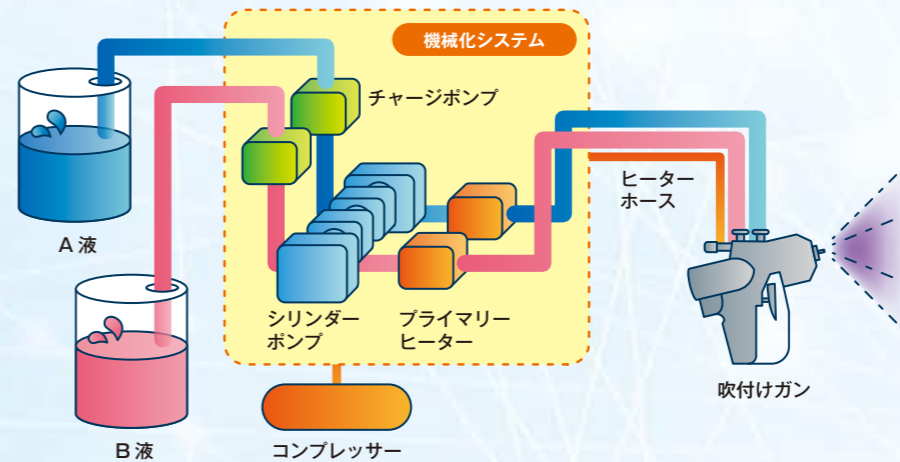
スプレーシステム概略図【例】
